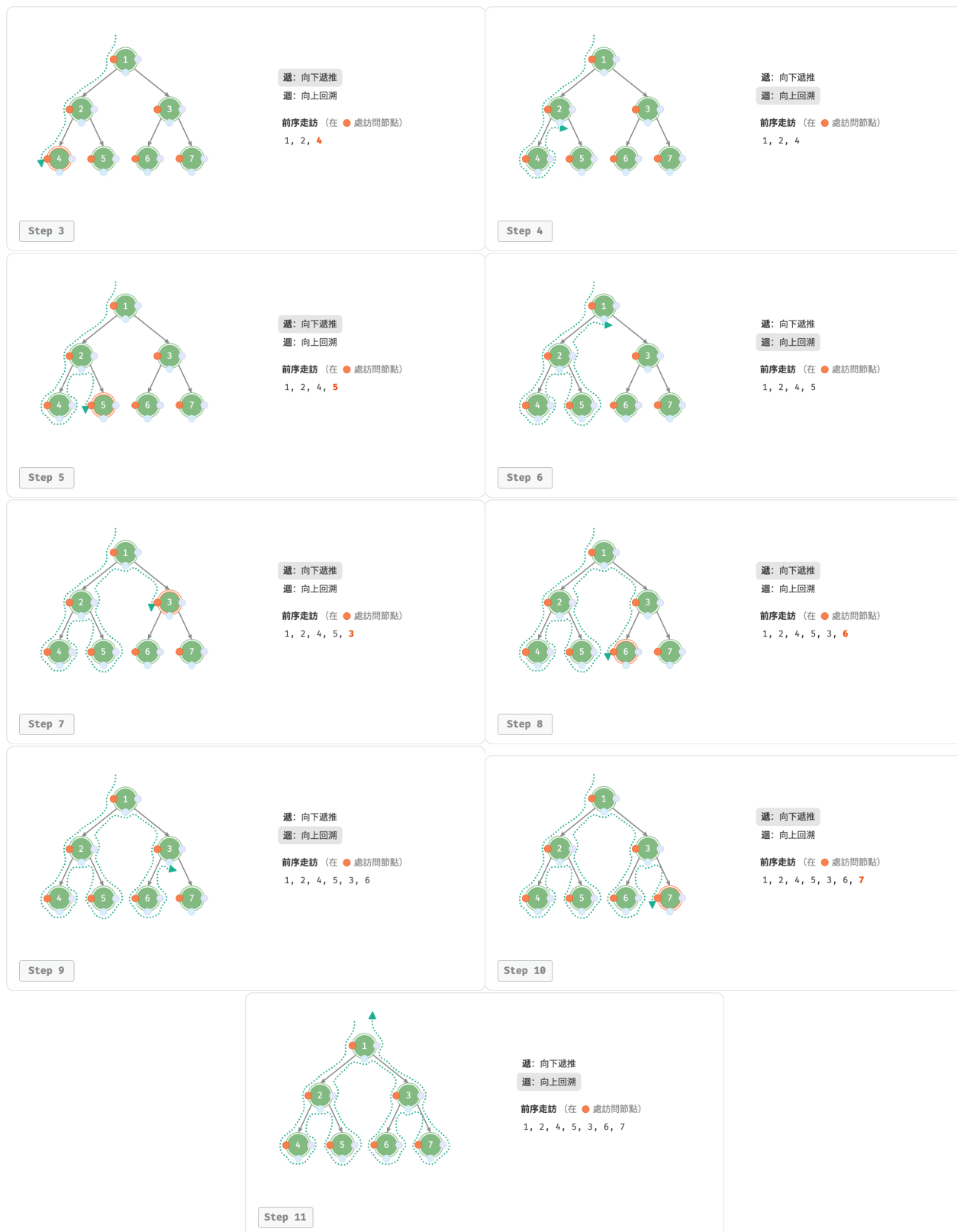
圖 7-11 前序走訪的遞迴過程
