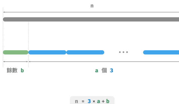
圖 15-16 最大切分乘積的計算方法
