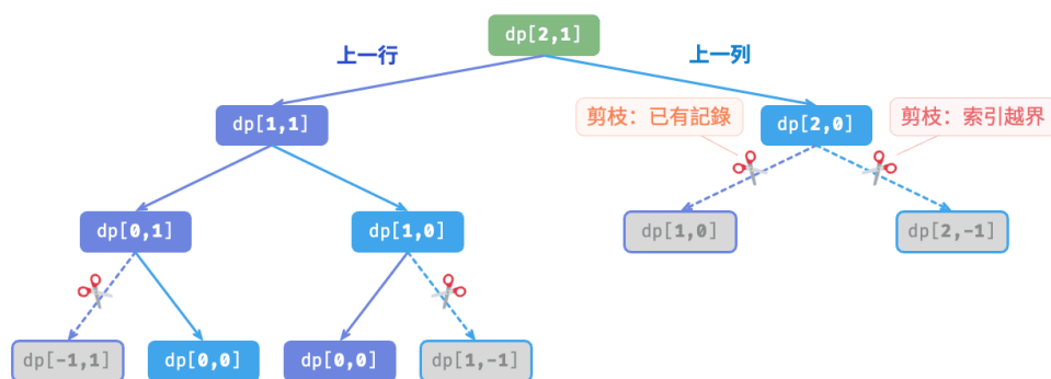
圖 14-15 記憶化搜尋遞迴樹
