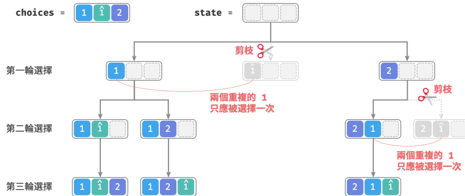
圖 13-8 重複排列剪枝
