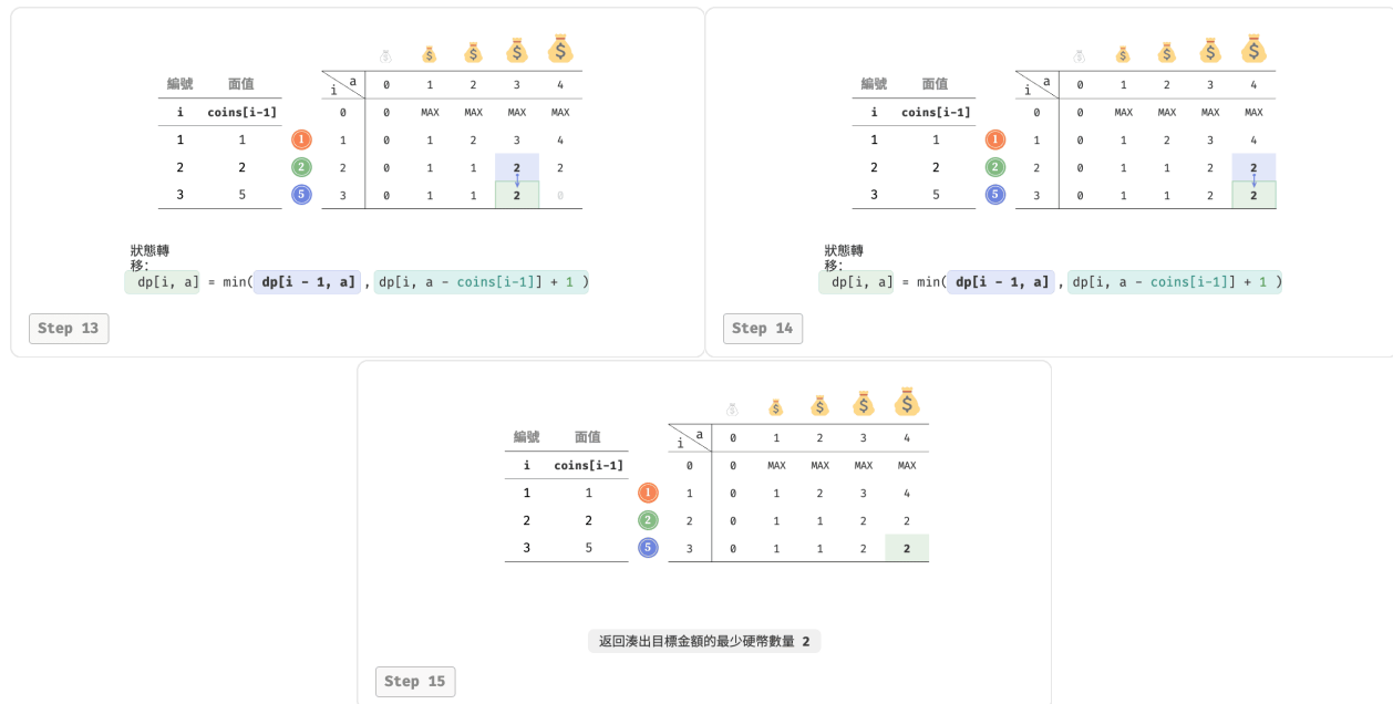
圖 14-25 零錢兌換問題的動態規劃過程
