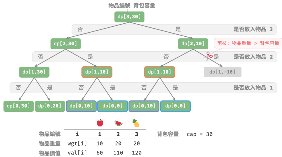
圖 14-18 0-1 背包問題的暴力搜尋遞迴樹
