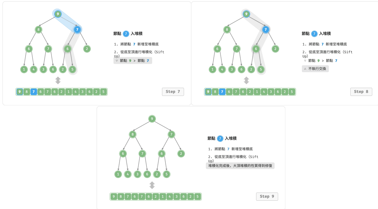
圖 8-3 元素入堆積步驟
