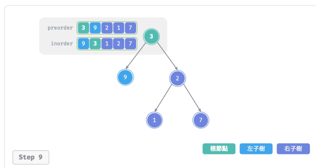
圖 12-8 構建二元樹的遞迴過程
