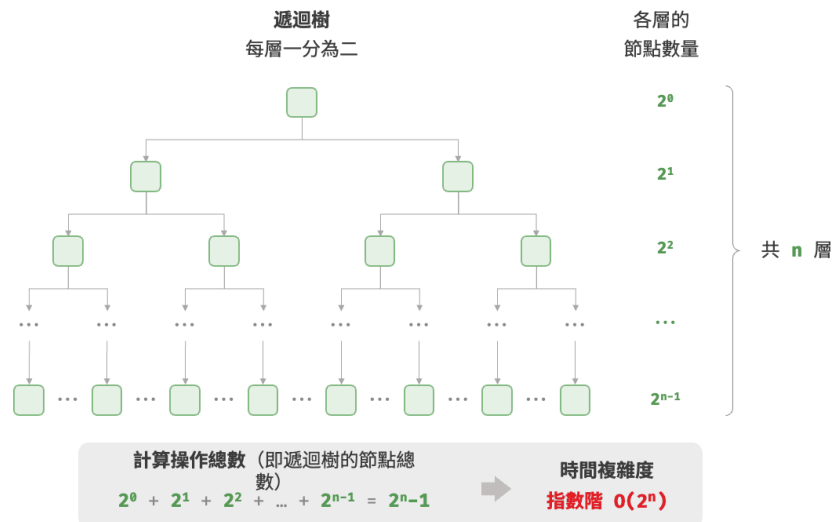
圖 2-11 指數階的時間複雜度
