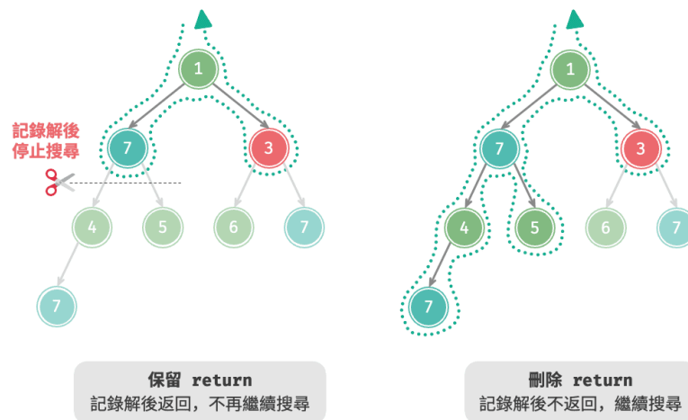
圖 13-4 保留與刪除 return 的搜尋過程對比
