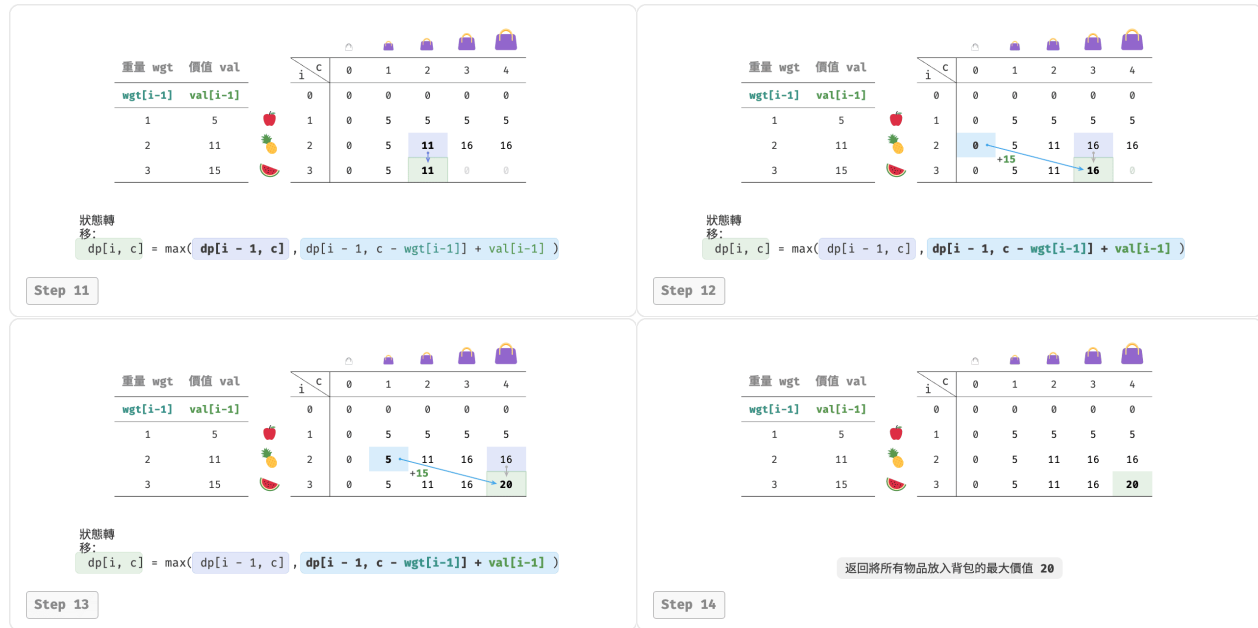
圖 14-20 0-1 背包問題的動態規劃過程
