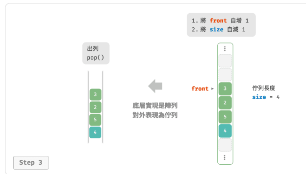
圖 5-6 基於陣列實現佇列的入列出列操作
