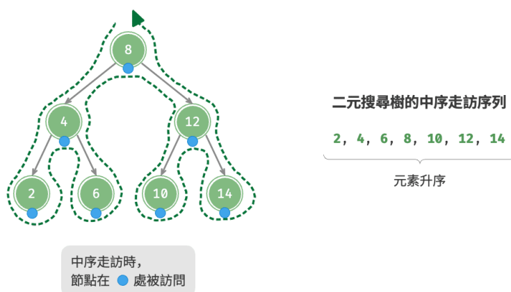
圖 7-22 二元搜尋樹的中序走訪序列
