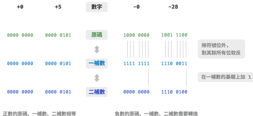
圖 3-4 原碼、一補數與二補數之間的相互轉換
