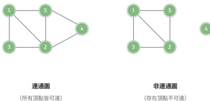
圖 9-3 連通圖與非連通圖
