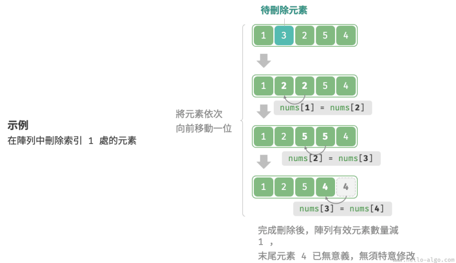
圖 4-4 陣列刪除元素示例
