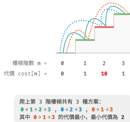
圖 14-6 爬到第 3 階的最小代價
