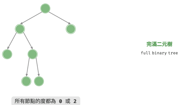
圖 7-6 完滿二元樹
