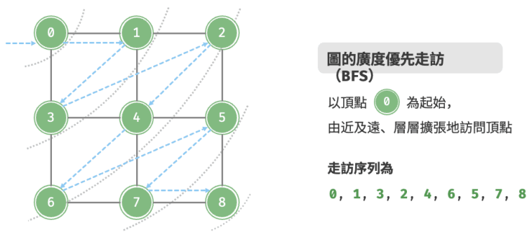
圖 9-9 圖的廣度優先走訪
