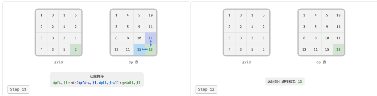
圖 14-16 最小路徑和的動態規劃過程
