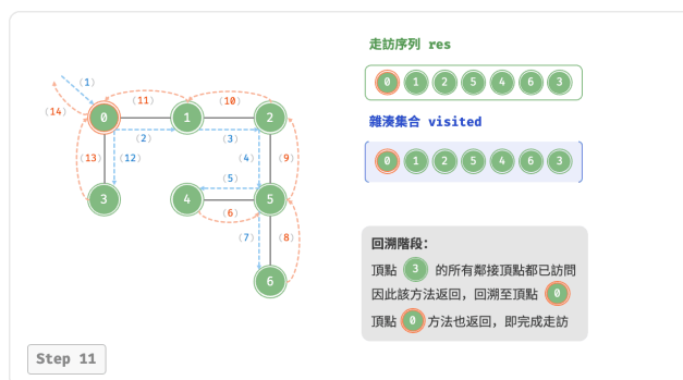
圖 9-12 圖的深度優先走訪步驟
