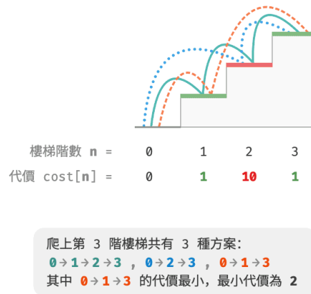
圖 14-6 爬到第 3 階的最小代價
