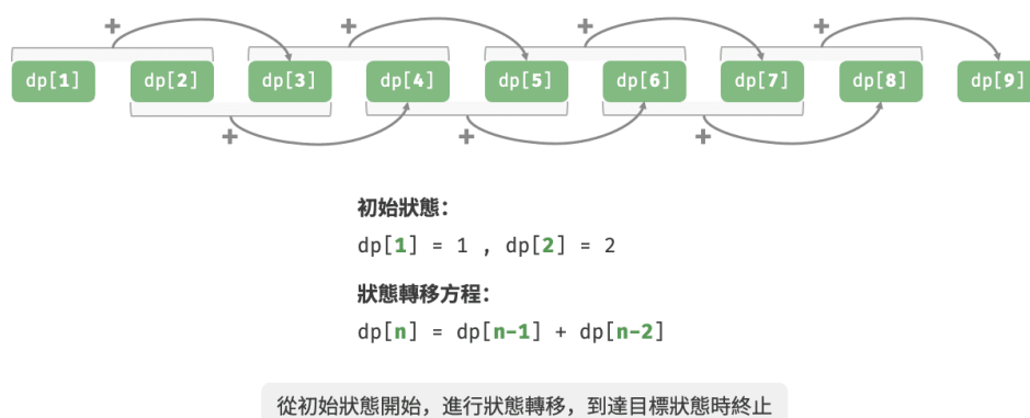
圖 14-5 爬樓梯的動態規劃過程
