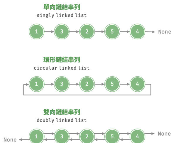
圖 4-8 常見鏈結串列種類
