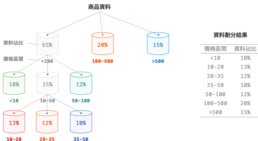
圖 11-14 遞迴劃分桶
