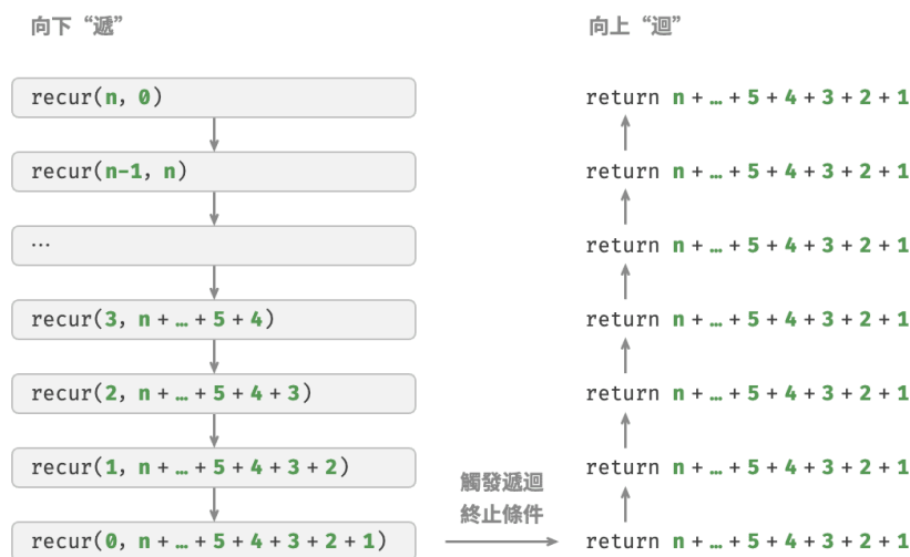
圖 2-5 尾遞迴過程
