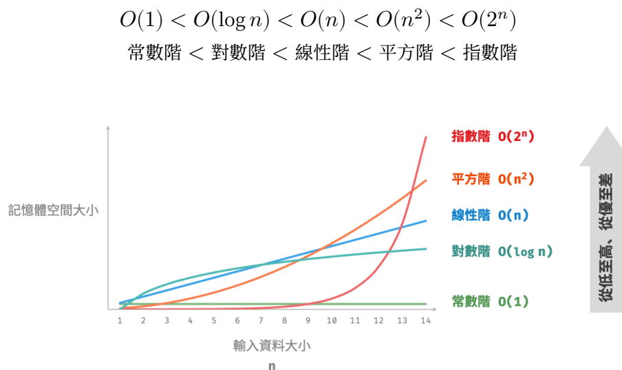
圖 2-16 常見的空間複雜度型別
