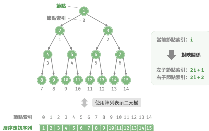
圖 7-12 完美二元樹的陣列表示
