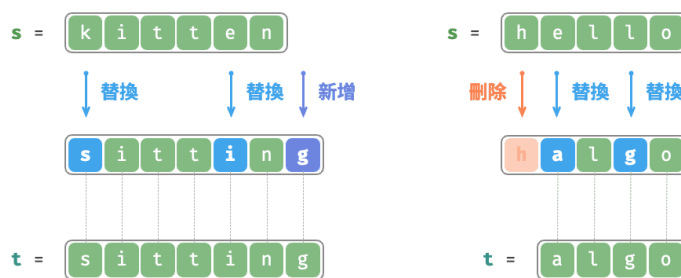
圖 14-27 編輯距離的示例資料
