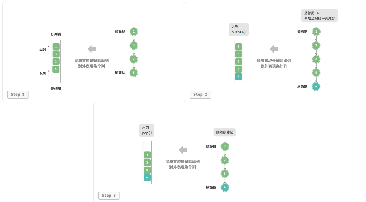
圖 5-5 基於鏈結串列表實現佇列的入列出列操作
