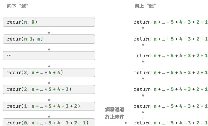
圖 2-5 尾遞迴過程
