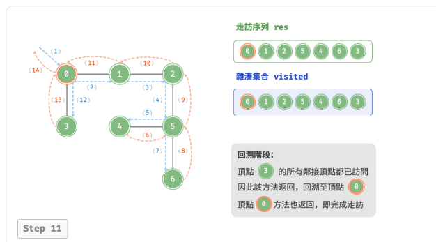
圖 9-12 圖的深度優先走訪步驟
