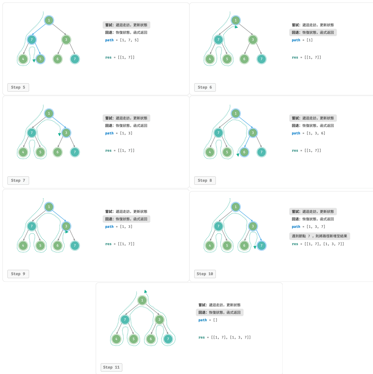
圖 13-2 嘗試與回退
