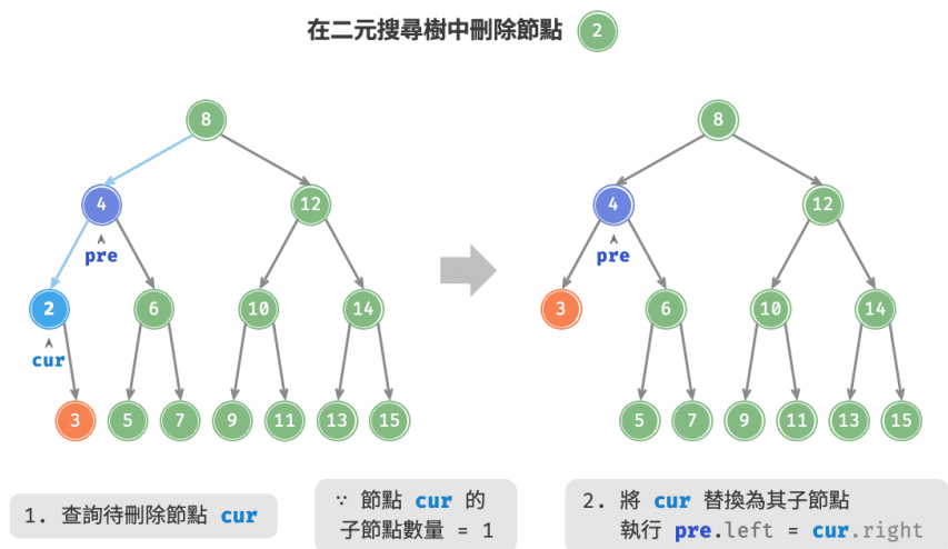
圖 7-20 在二元搜尋樹中刪除節點（度為 1）
