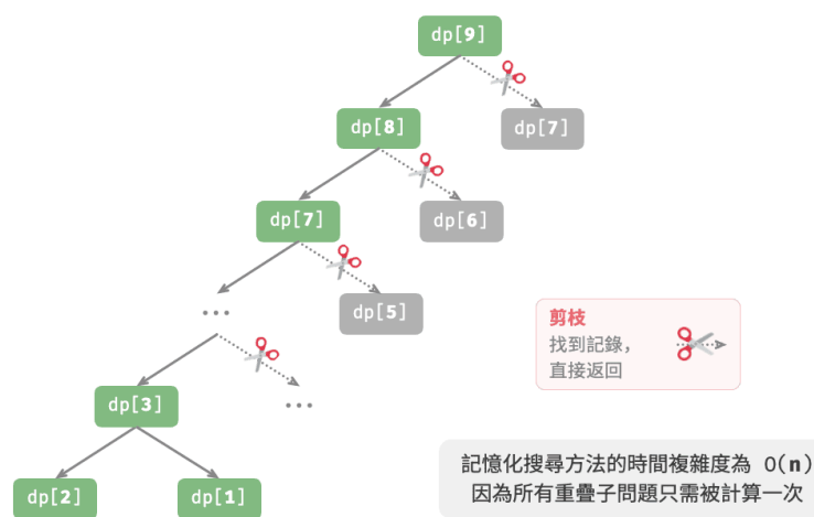
圖 14-4 記憶化搜尋對應遞迴樹
