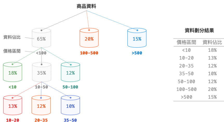
圖 11-14 遞迴劃分桶
