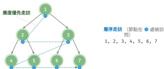
圖 7-9 二元樹的層序走訪
