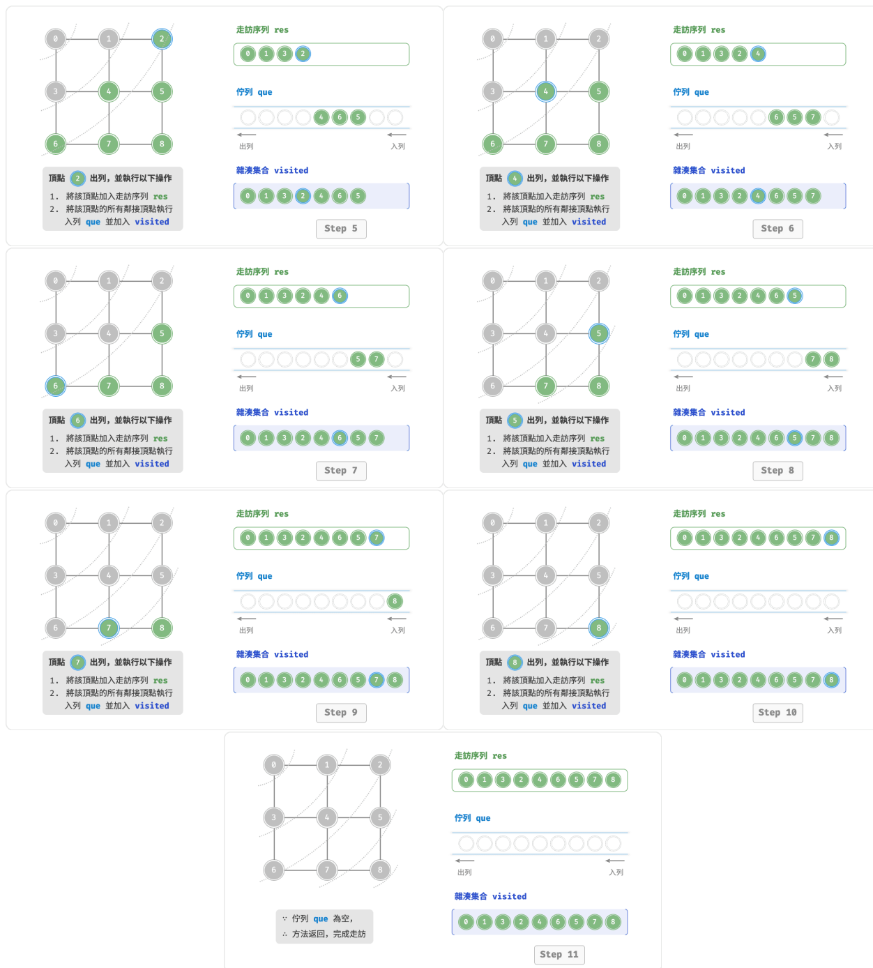
圖 9-10 圖的廣度優先走訪步驟
