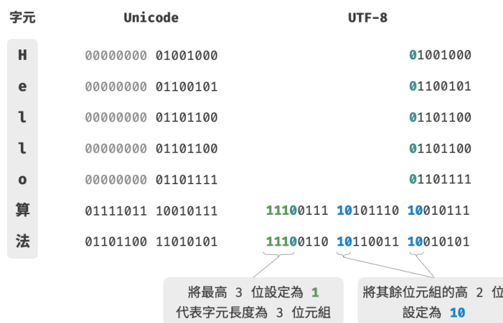
圖 3-8 UTF-8 編碼示例
