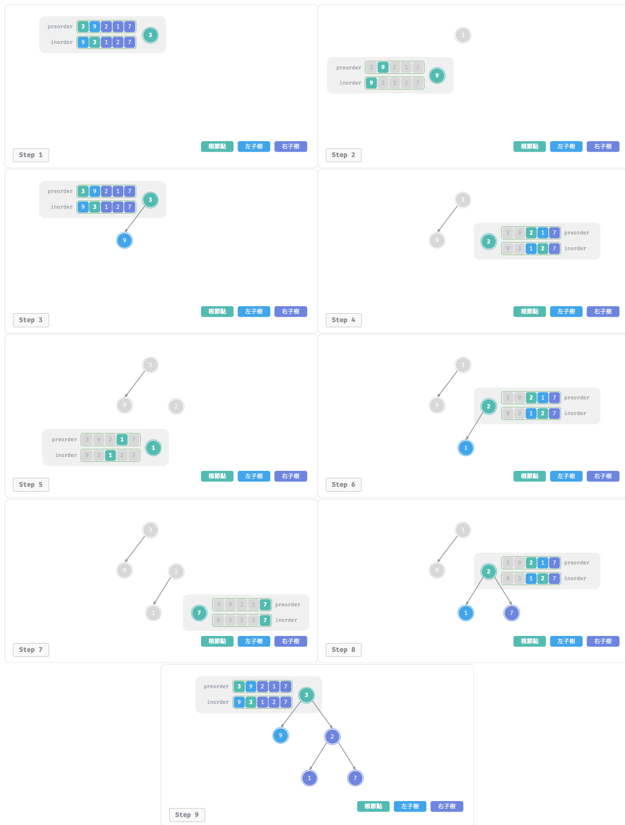
圖 12-8 構建二元樹的遞迴過程
