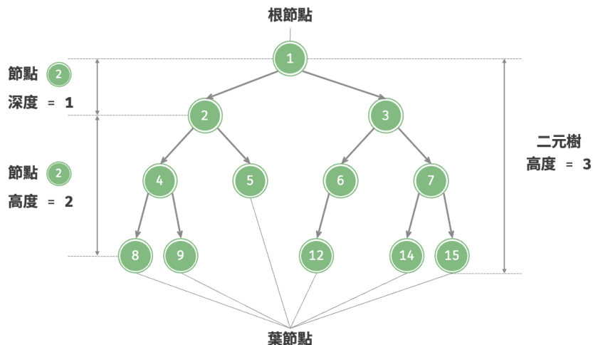
圖 7-2 二元樹的常用術語
