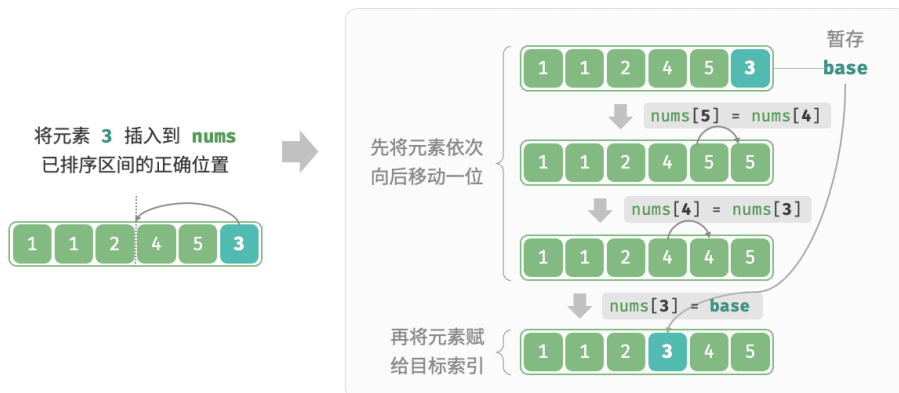
图 11-6 单次插入操作
