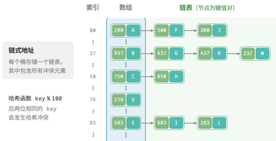
图 6-5 链式地址哈希表
