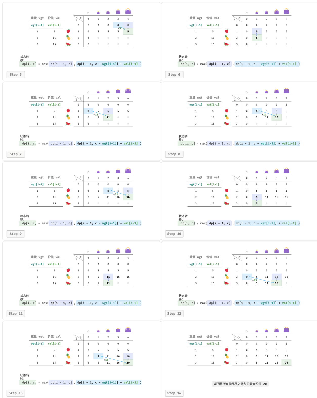
图 14-20 0-1 背包问题的动态规划过程
