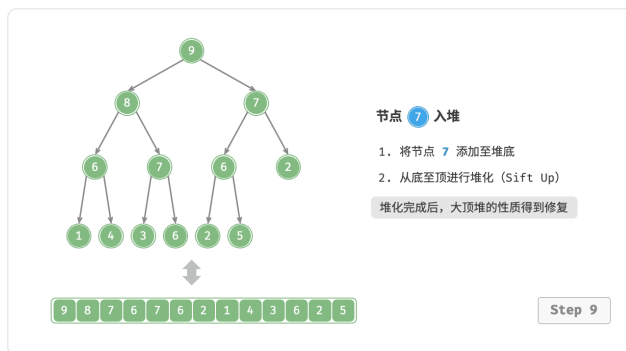
图 8-3 元素入堆步骤
