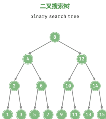
图 7-16 二叉搜索树
