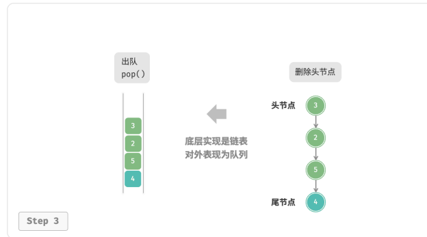
图 5-5 基于链表实现队列的入队出队操作
