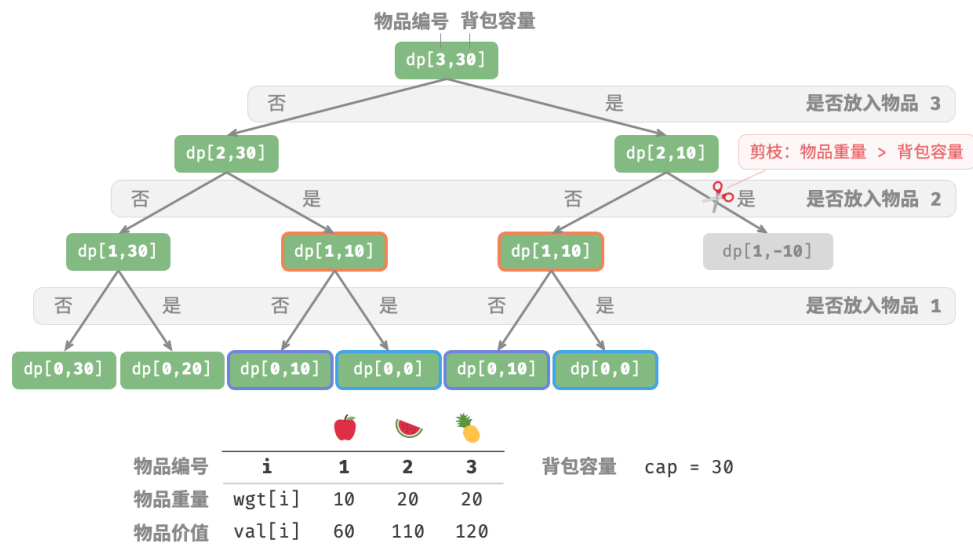
图 14-18 0-1 背包问题的暴力搜索递归树
