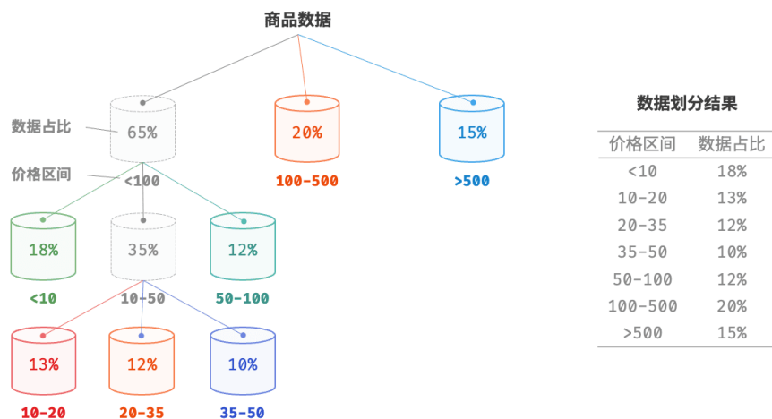
图 11-14 递归划分桶
