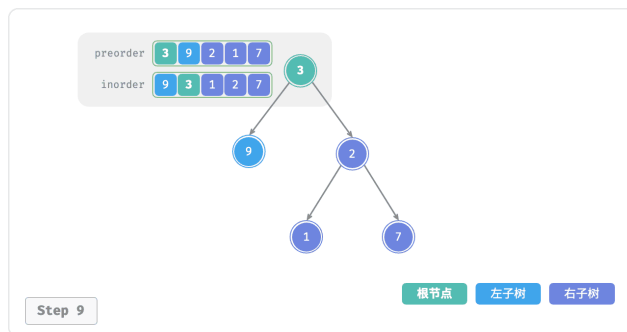
图 12-8 构建二叉树的递归过程
