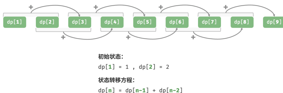
图 14-5 模拟了以上代码的执行过程。
