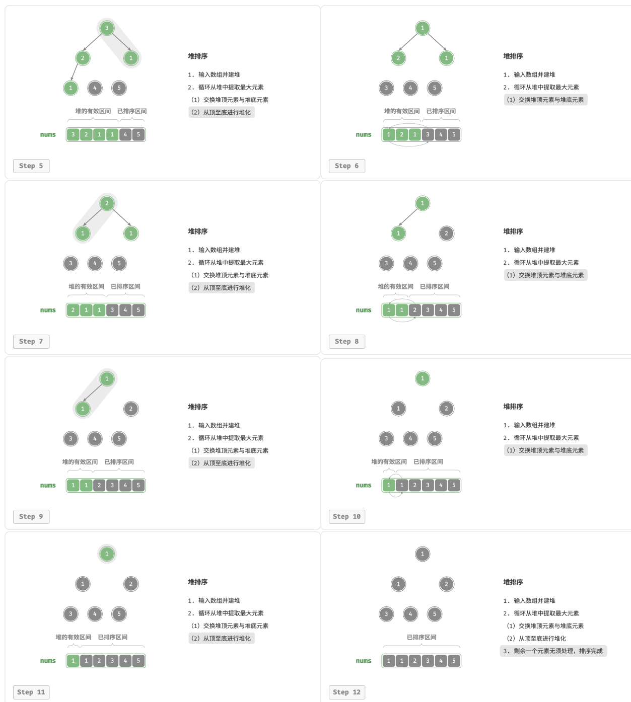
图 11-12 堆排序步骤
