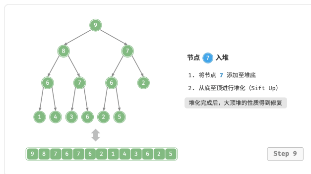
图 8-3 元素入堆步骤
