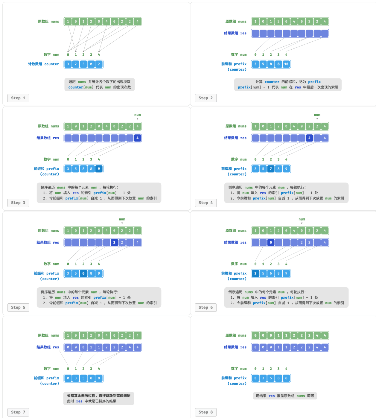
图 11-17 计数排序步骤
