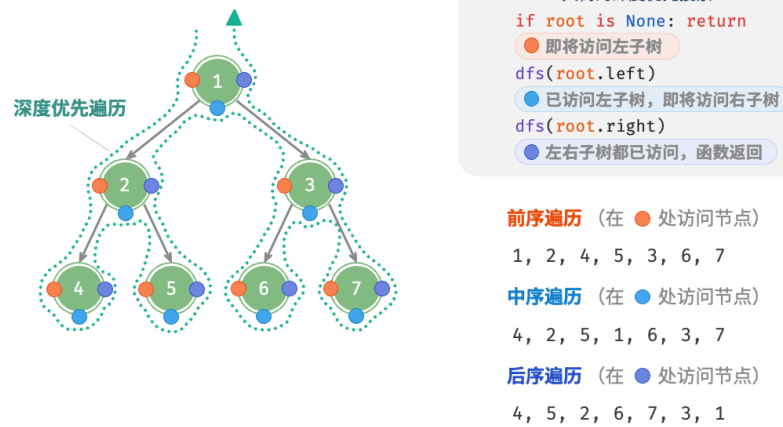
图 7-10 二叉搜索树的前序、中序、后序遍历
