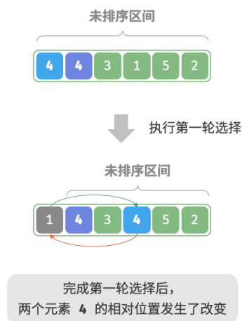
图 11-3 选择排序非稳定示例
