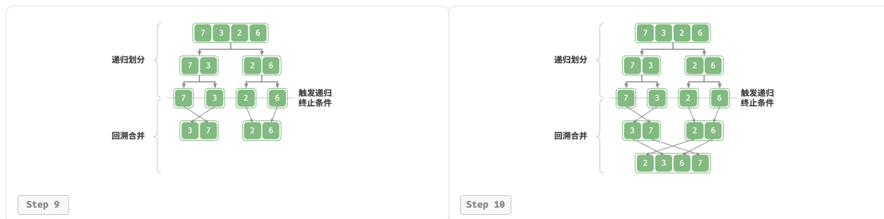
图 11-11 归并排序步骤
