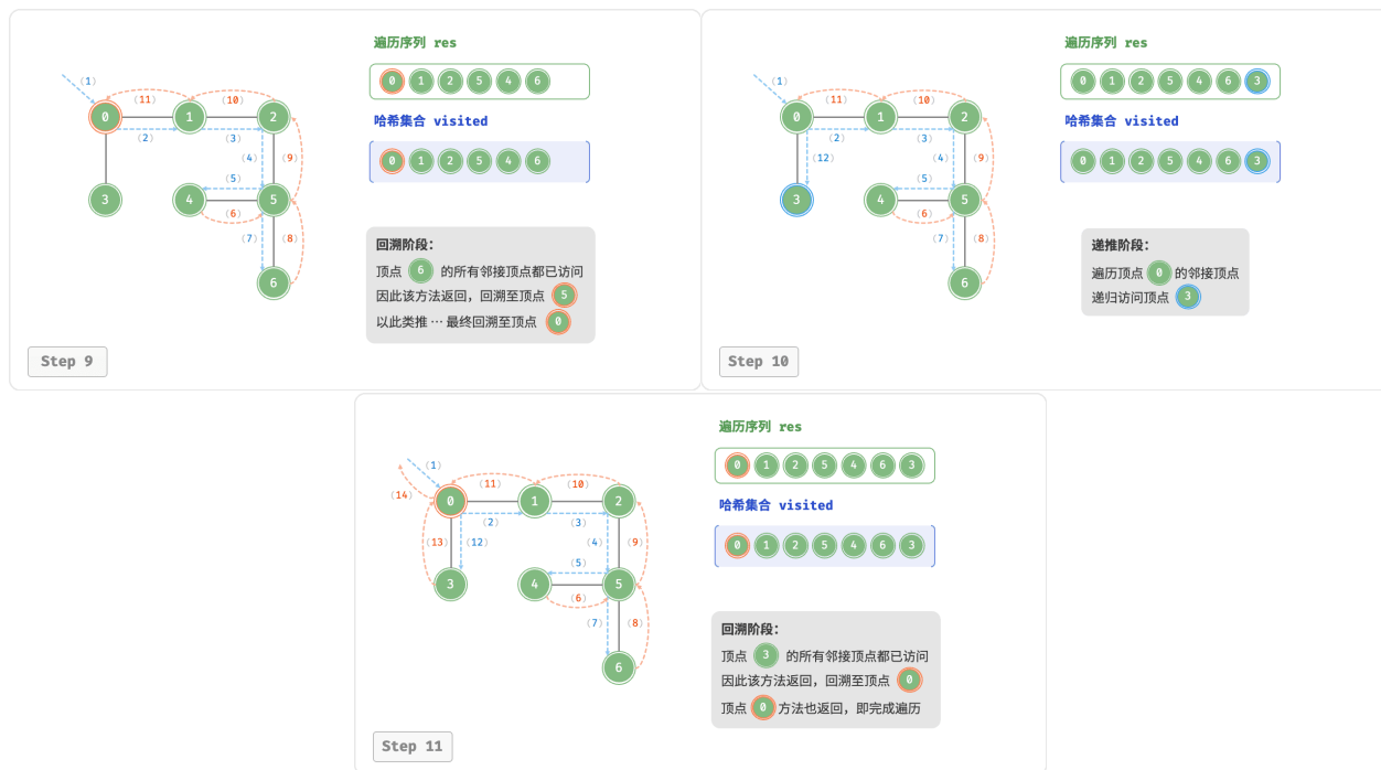
图 9-12 图的深度优先遍历步骤
