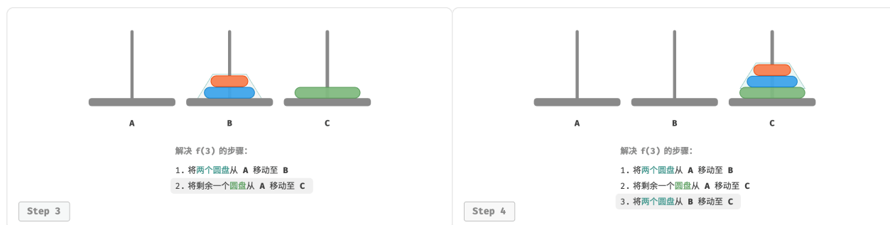
图 12-13 规模为 3 的问题的解
