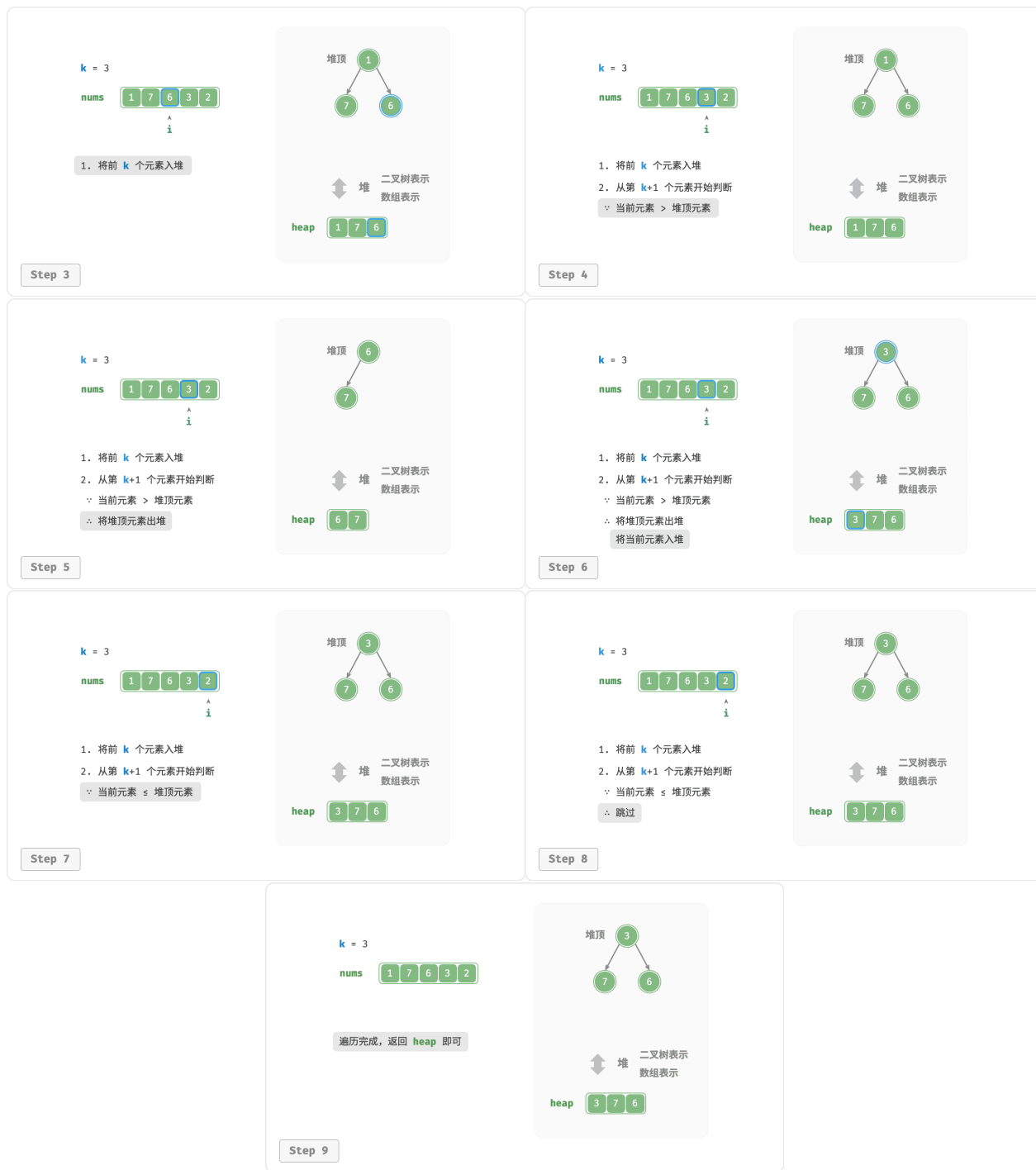
图 8-8 基于堆寻找最大的 k 个元素
