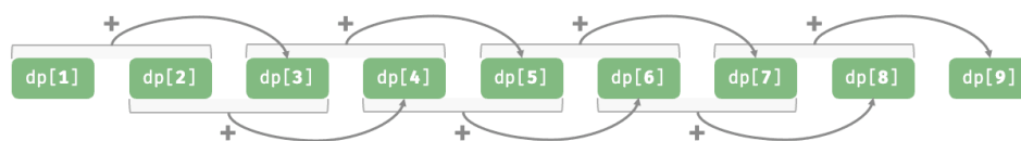
图 14-5 模拟了以上代码的执行过程。
