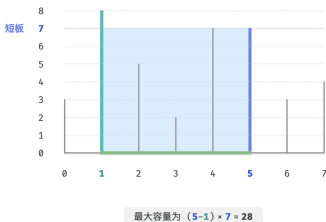
图 15-7 最大容量问题的示例数据
