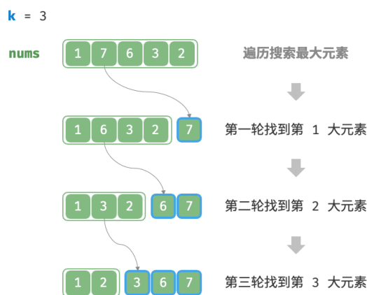
图 8-6 遍历寻找最大的 k 个元素
