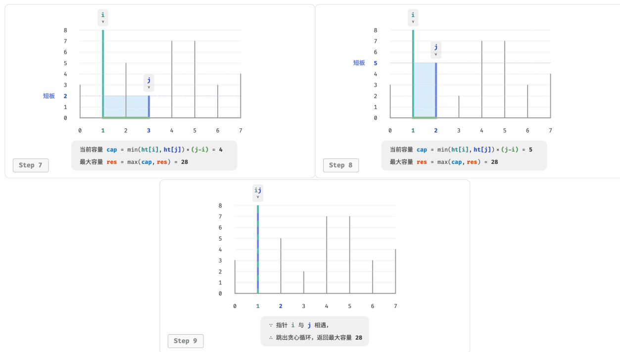
图 15-11 最大容量问题的贪心过程
