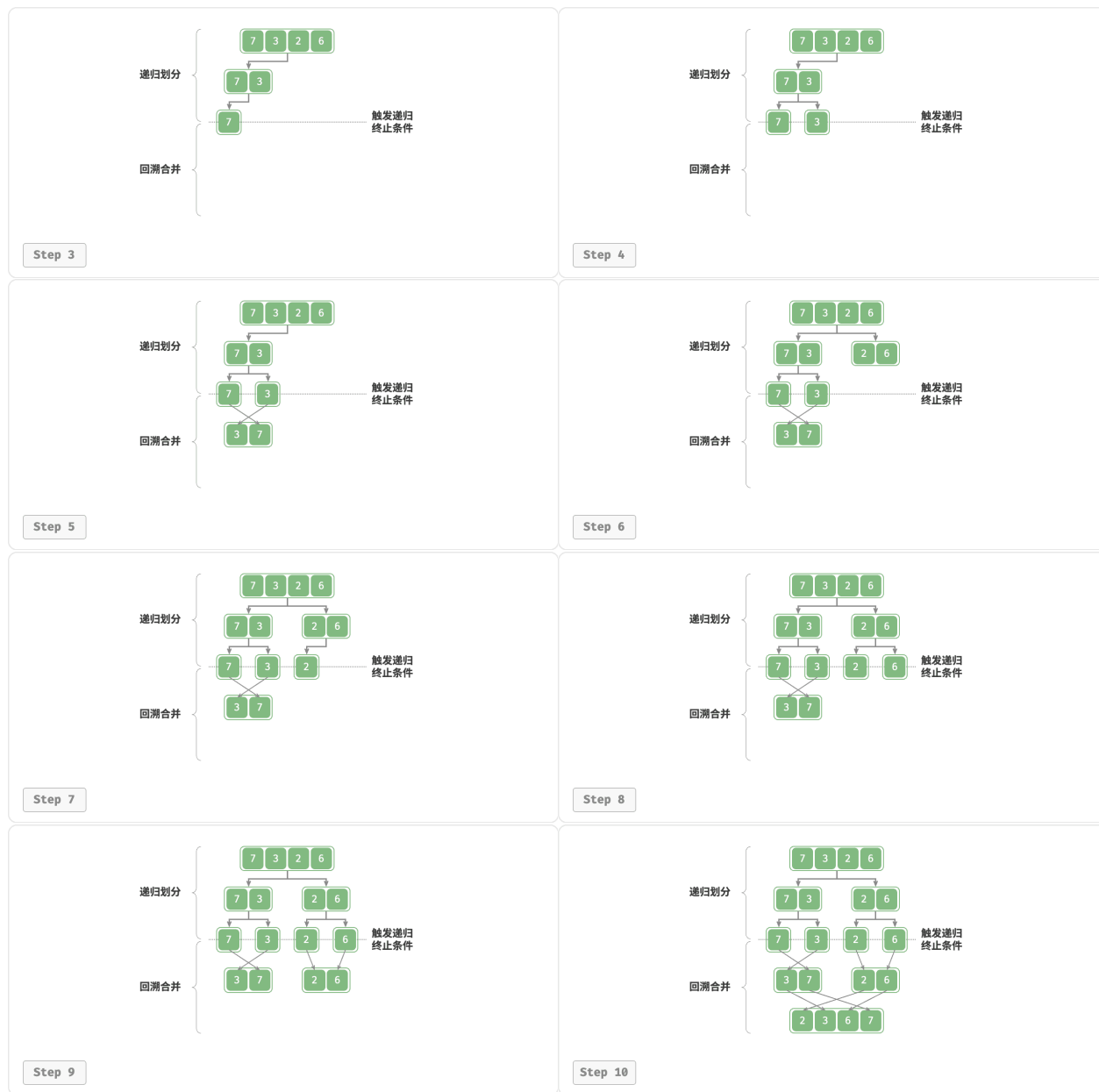
图 11-11 归并排序步骤
