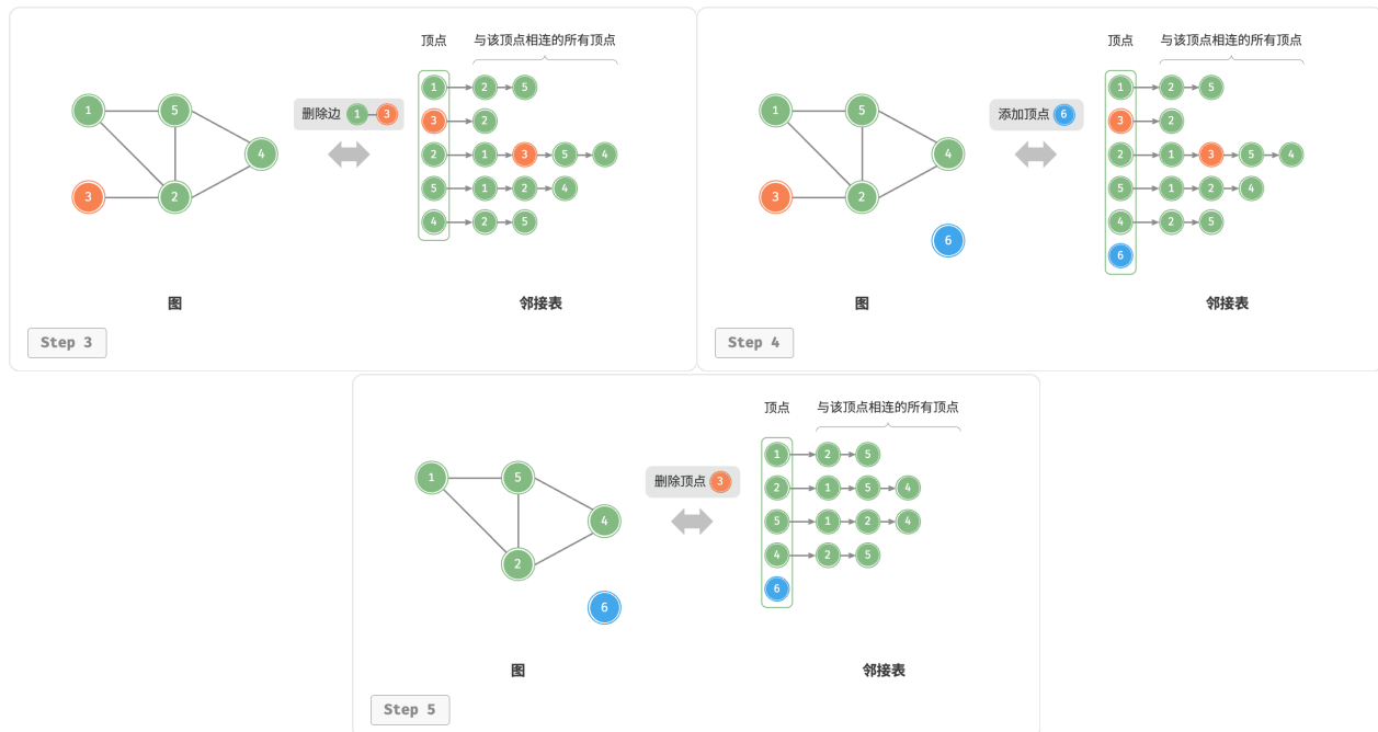
图 9-8 邻接表的初始化、增删边、增删顶点
