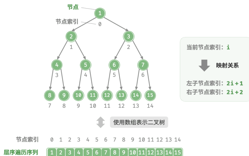
图 7-12 完美二叉树的数组表示
