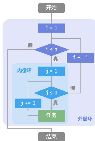
图 2-2 嵌套循环的流程框图
