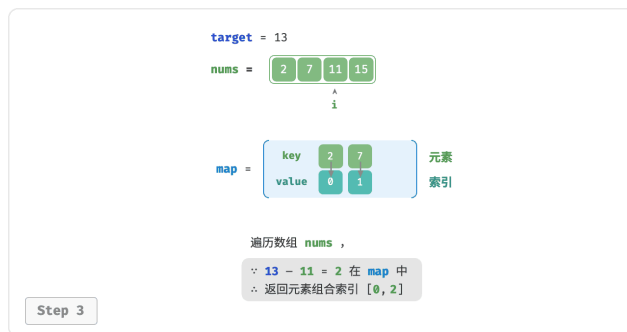
图 10-10 辅助哈希表求解两数之和
