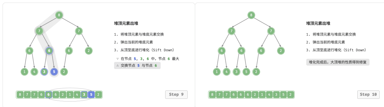
图 8-4 堆顶元素出堆步骤
