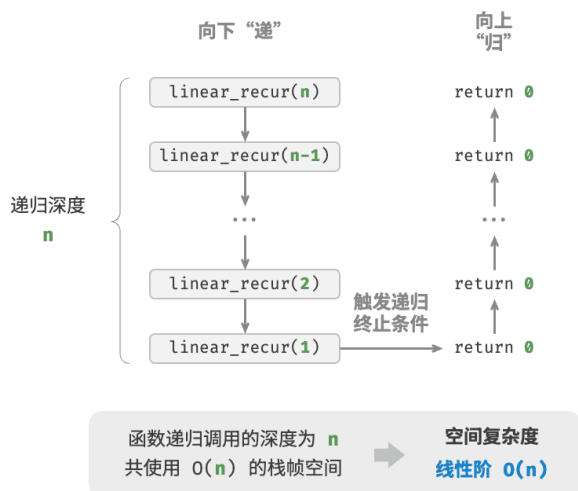
图 2-17 递归函数产生的线性阶空间复杂度
