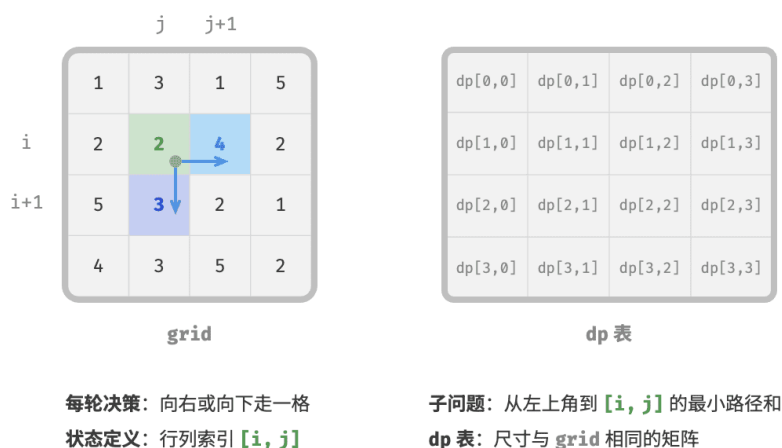
图 14-11 状态定义与 dp 表
