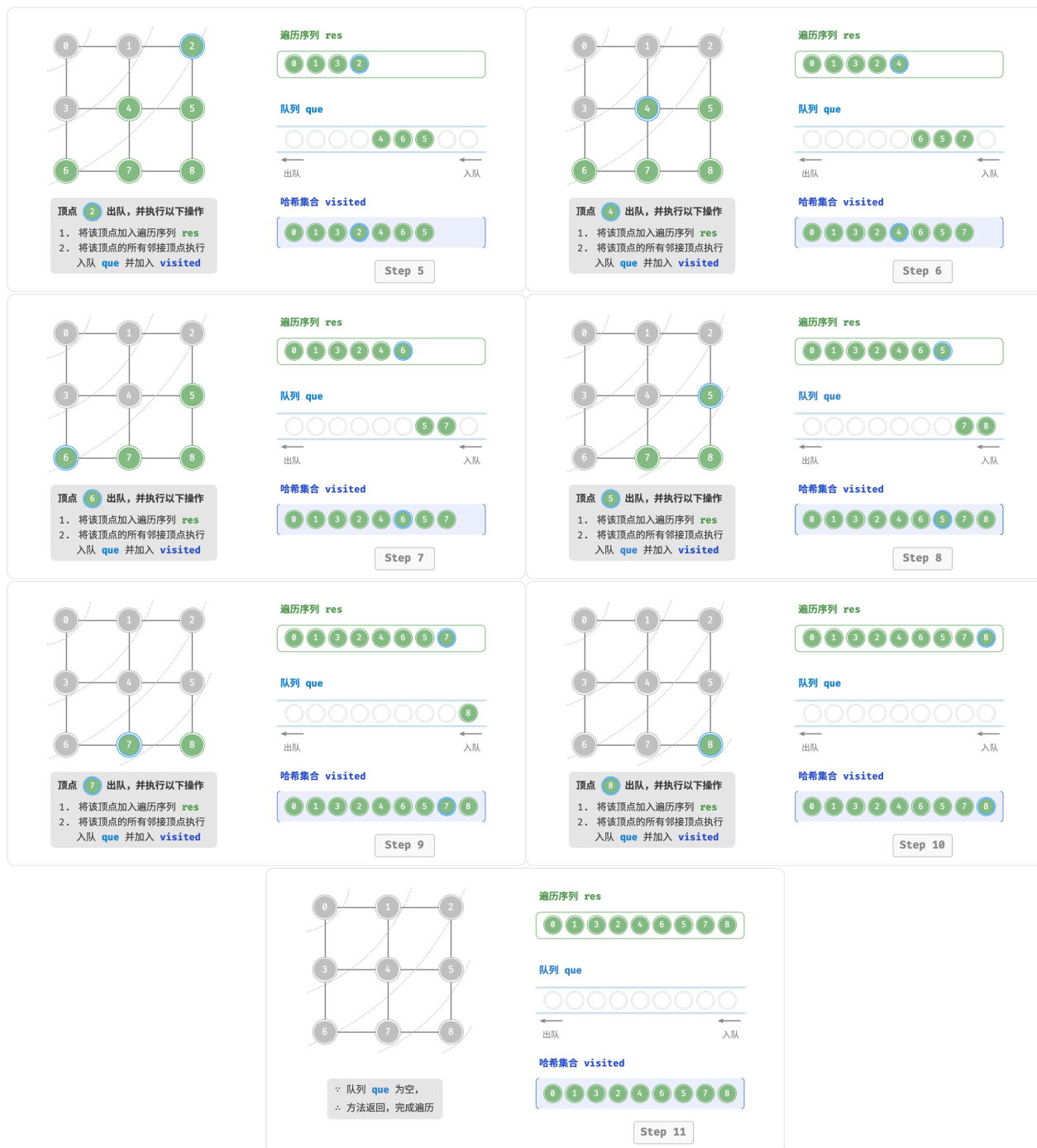
图 9-10 图的广度优先遍历步骤
