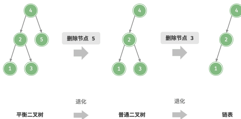
图 7-24 AVL 树在删除节点后发生退化
