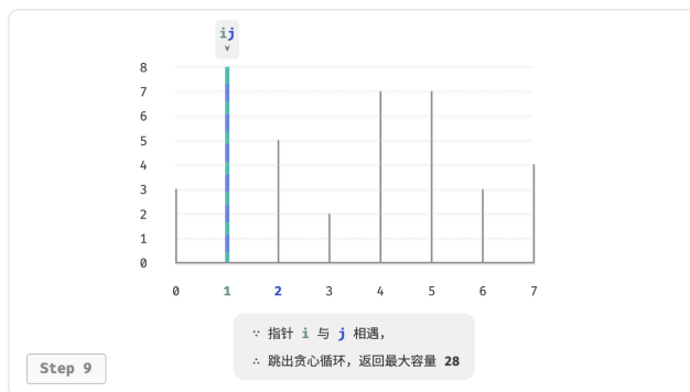
图 15-11 最大容量问题的贪心过程
