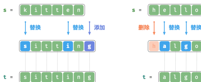
图 14-27 编辑距离的示例数据
