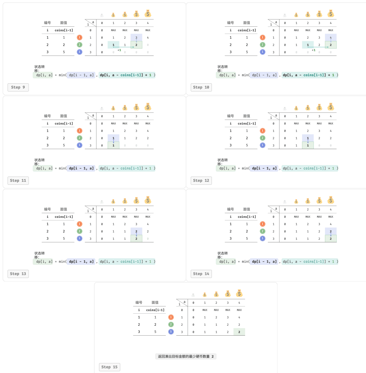
图 14-25 零钱兑换问题的动态规划过程
