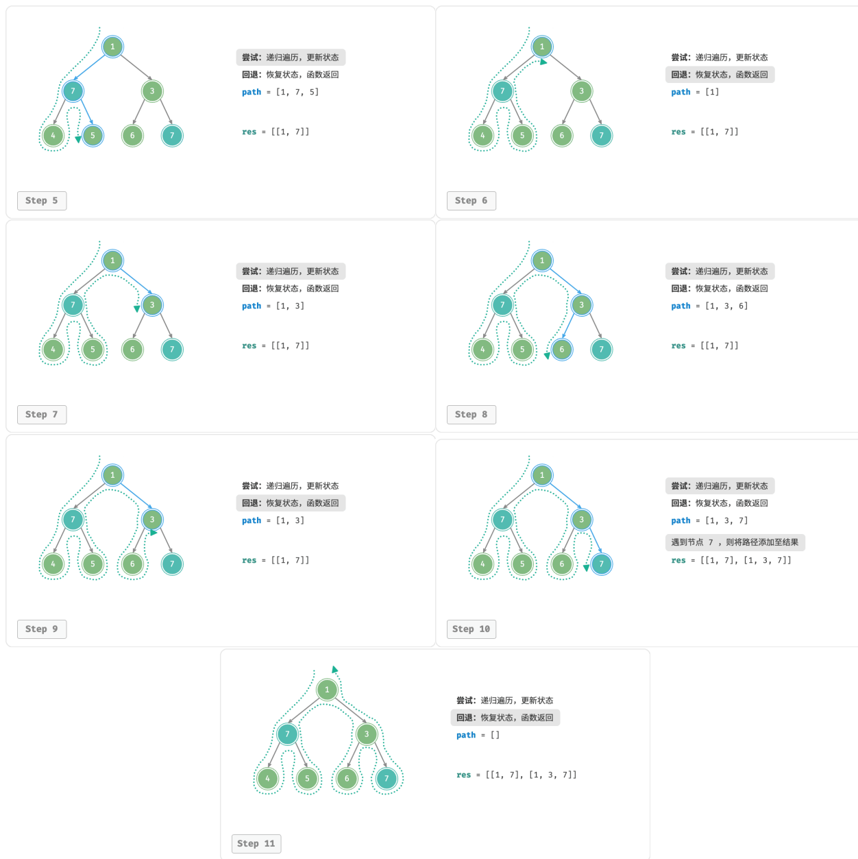
图 13-2 尝试与回退
