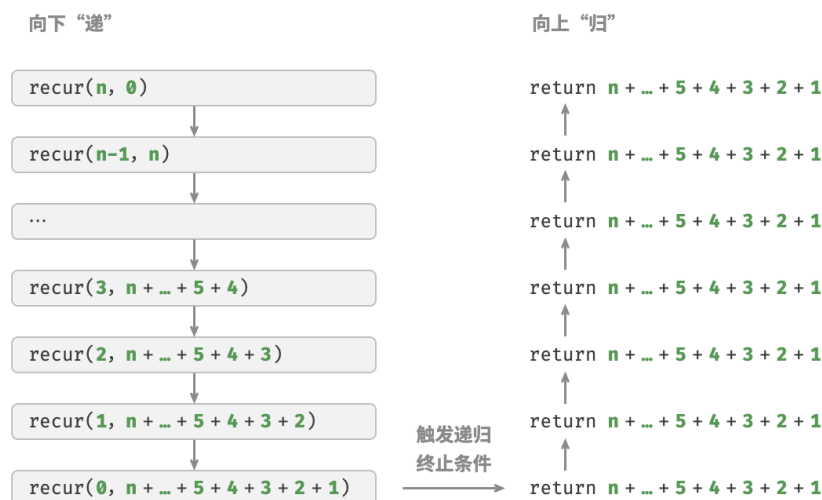
图 2-5 尾递归过程
