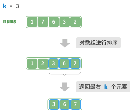
图 8-7 排序寻找最大的 k 个元素
