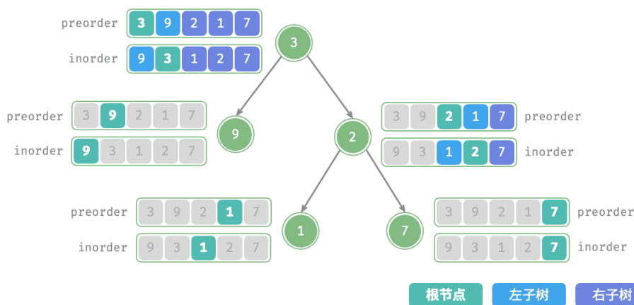
图 12-9 每个递归函数中的划分结果
