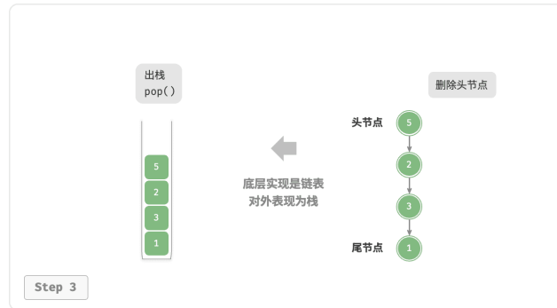
图 5-2 基于链表实现栈的入栈出栈操作
