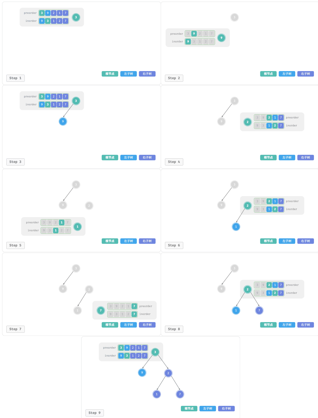
图 12-8 构建二叉树的递归过程
