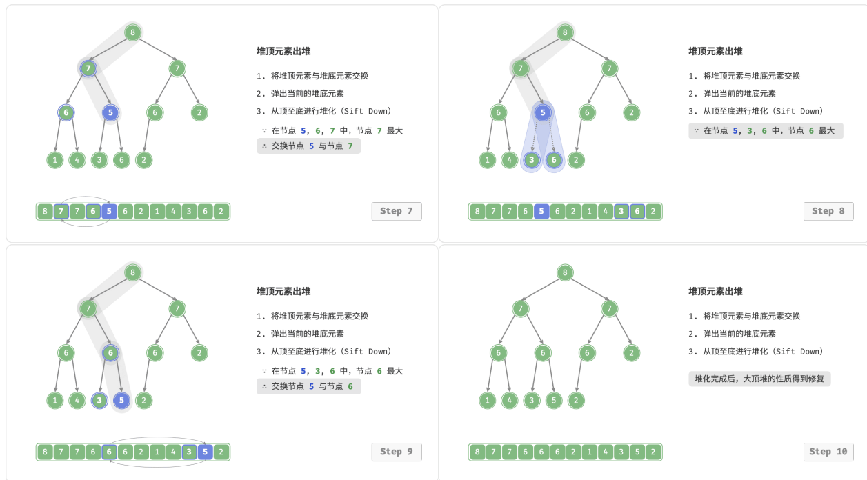
图 8-4 堆顶元素出堆步骤
