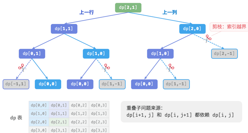
图 14-14 暴力搜索递归树
