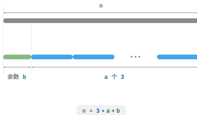
图 15-16 最大切分乘积的计算方法
