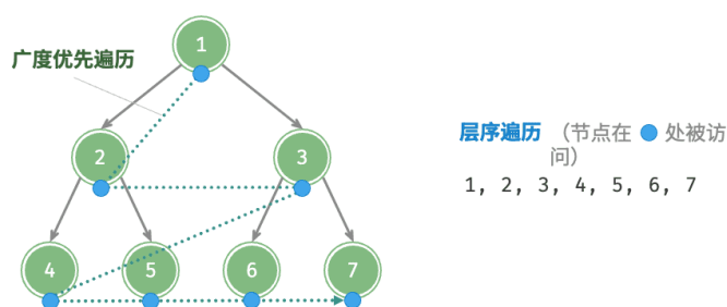
图 7-9 二叉树的层序遍历
