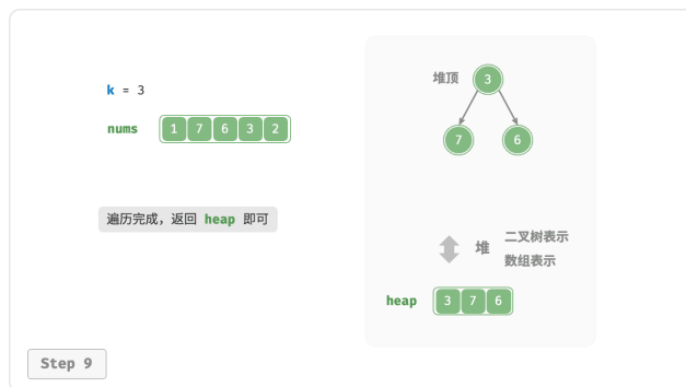
图 8-8 基于堆寻找最大的 k 个元素
