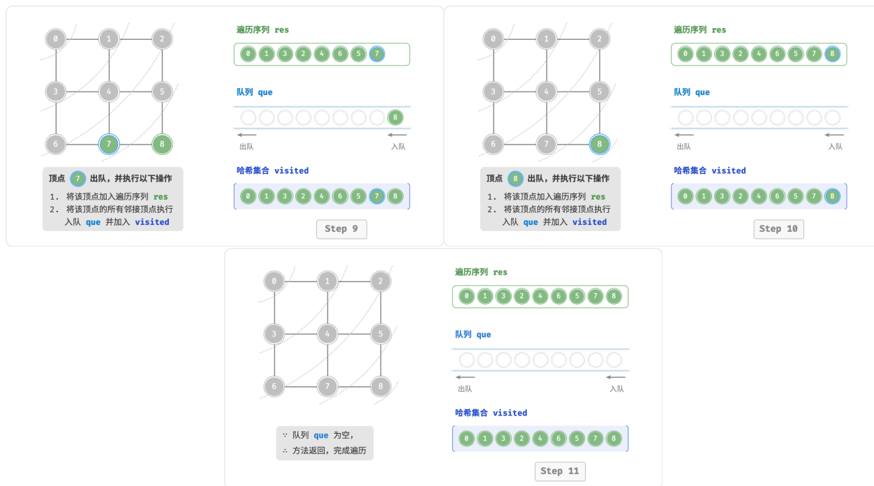
图 9-10 图的广度优先遍历步骤
