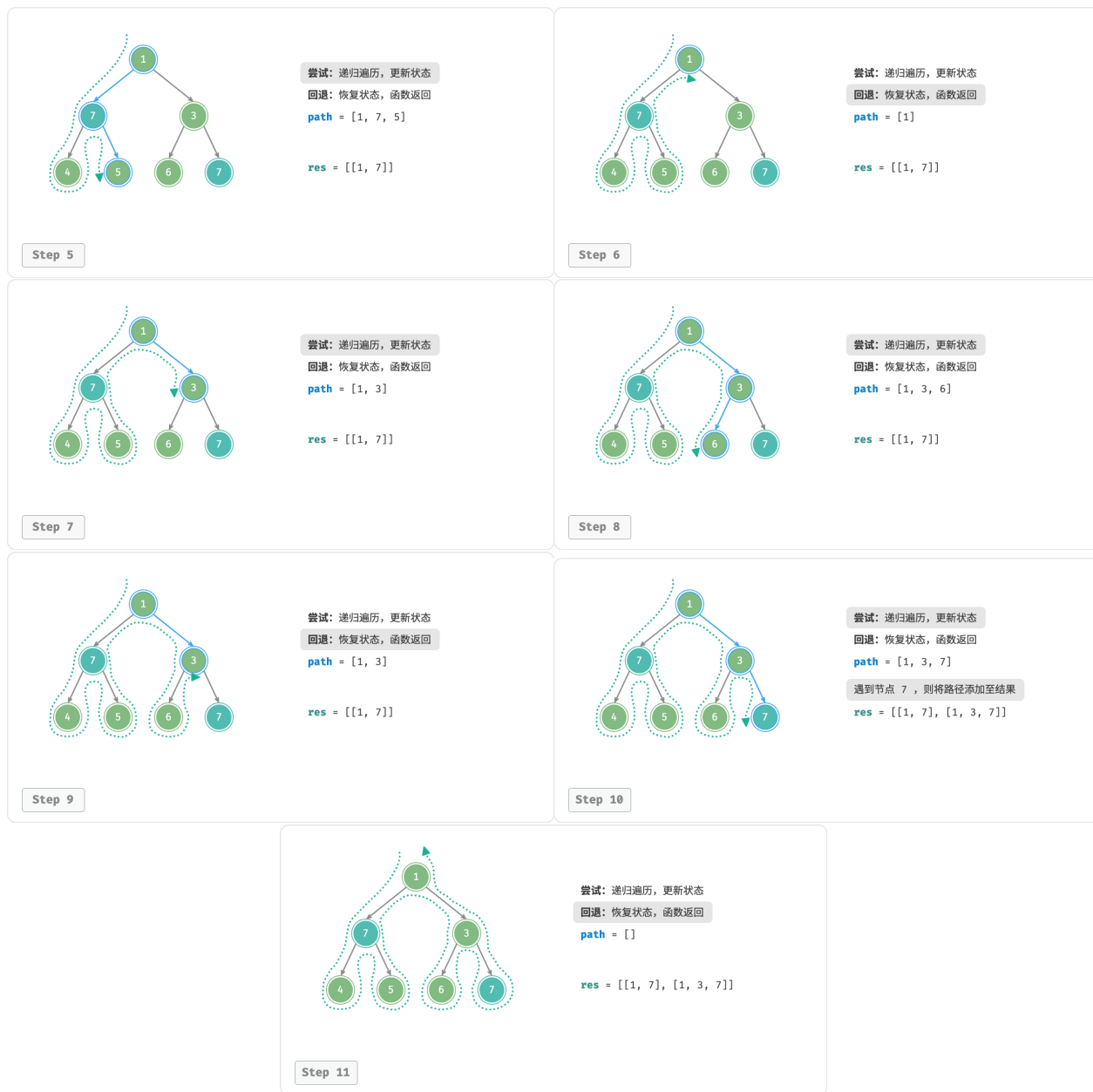
图 13-2 尝试与回退
