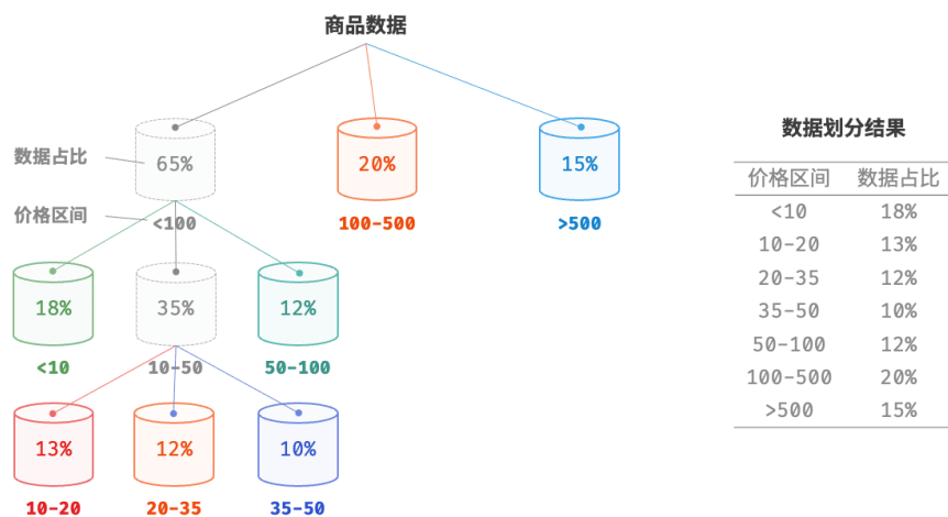
图 11-14 递归划分桶
