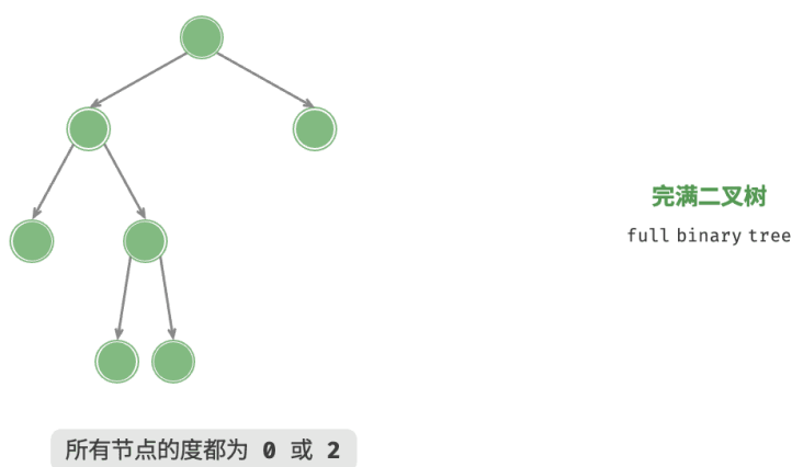
图 7-6 完满二叉树
