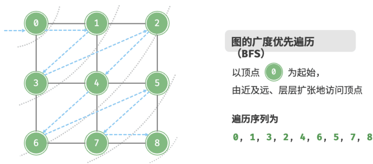
图 9-9 图的广度优先遍历
